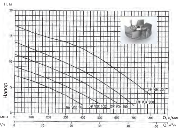
насосы с вихревым рабочим колесом
